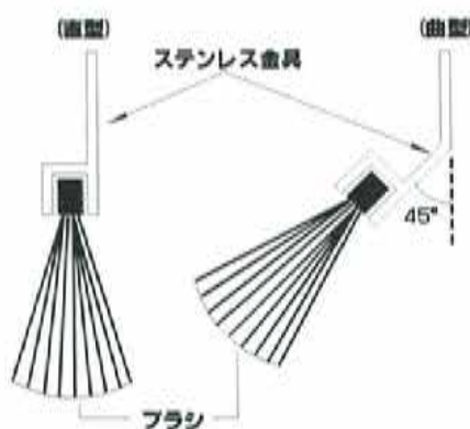
取り付け例
