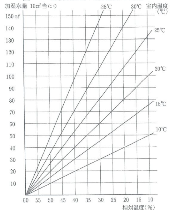
図-4 湿度調整用：加湿倍率早見表
